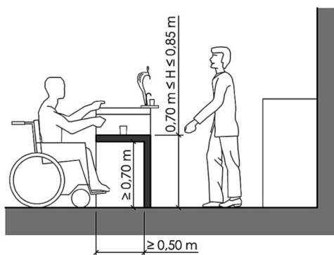
MOSTRADOR SECCIÓN
