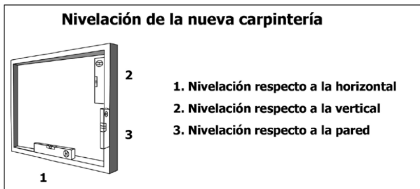
Figura 14. Nivelación de la nueva carpintería
